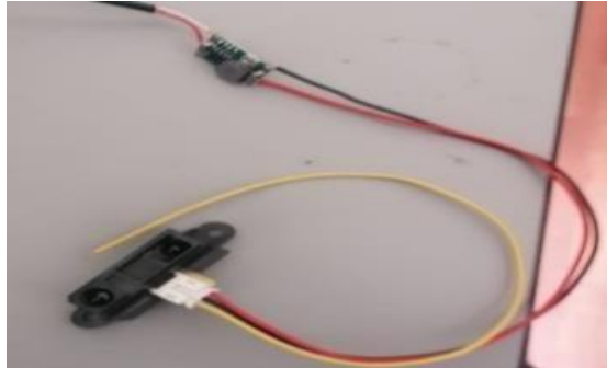
Figura 3. Sensor Sharp analógico de distancia GP2Y0A21YK0F.
